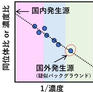
図 キーリングプロット 概念図
